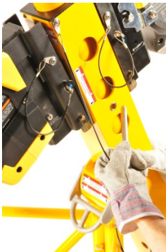
Fig. 24 Paso 8A
